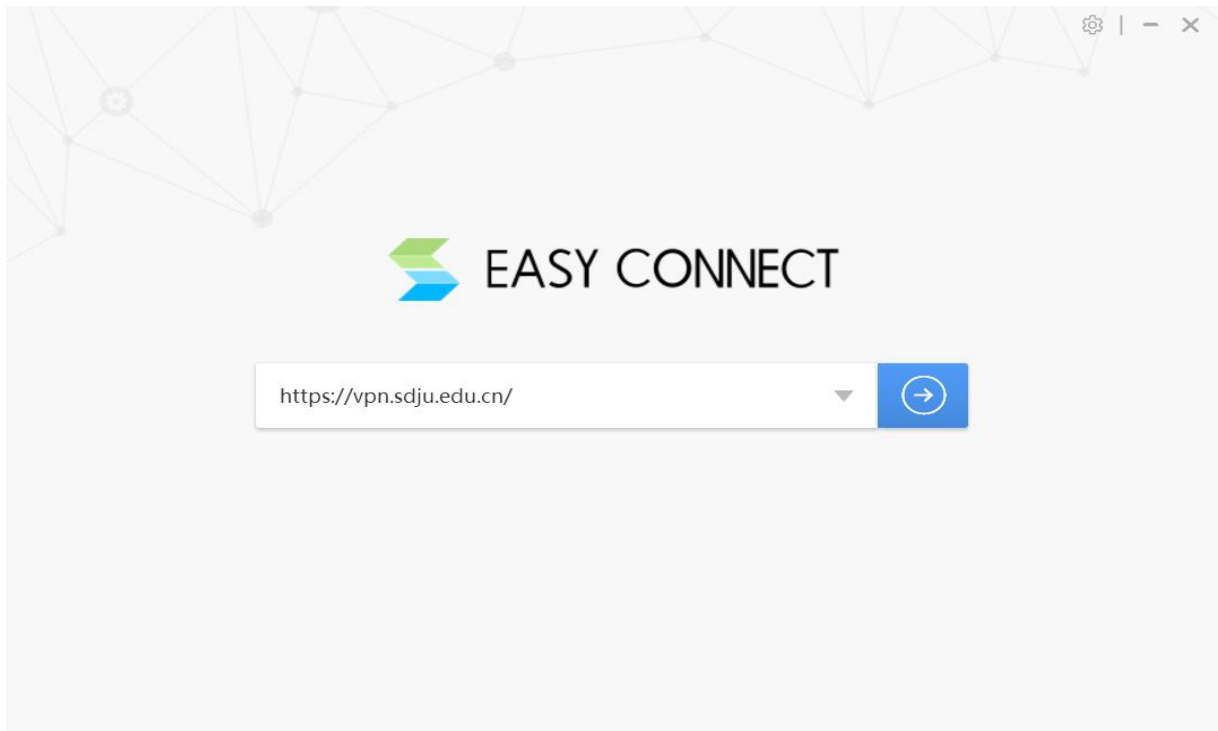
图 1.3 连接对话框
